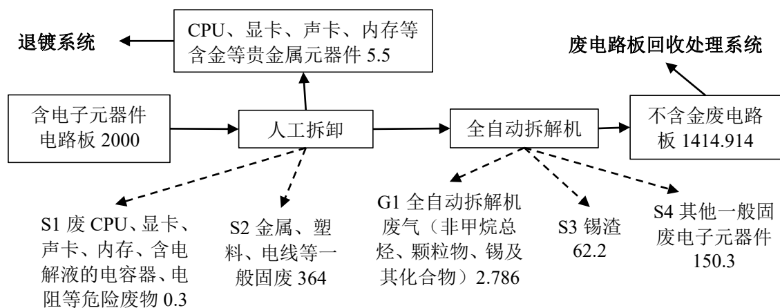
图 3.4-2 废电路板元器件拆解系统物料平衡图（单位 t/a）
