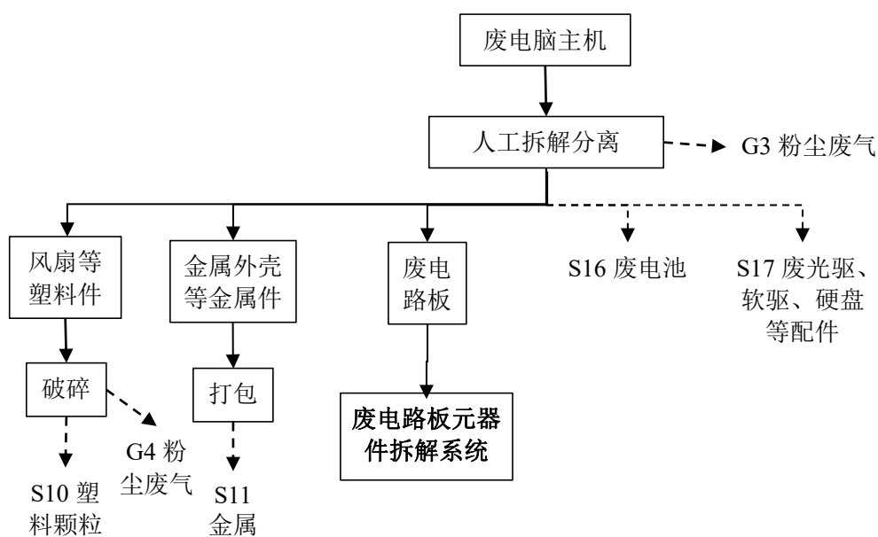
图 3.4-14 废电脑主机拆解工艺流程及产污环节图
