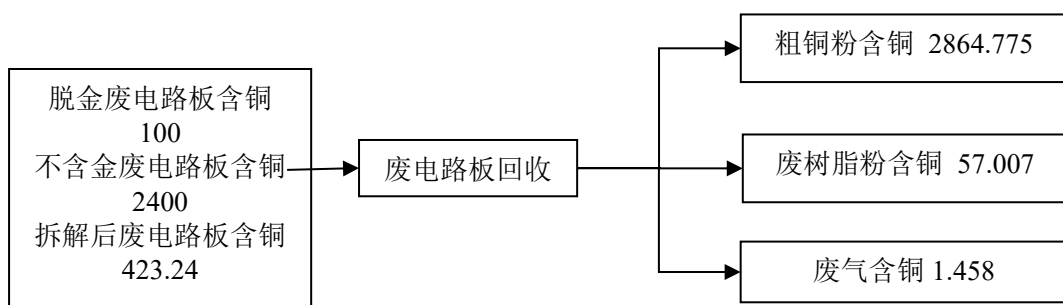
图 3.4-5 废电路板破碎分选生产线铜元素平衡示意图 单位: t/a
