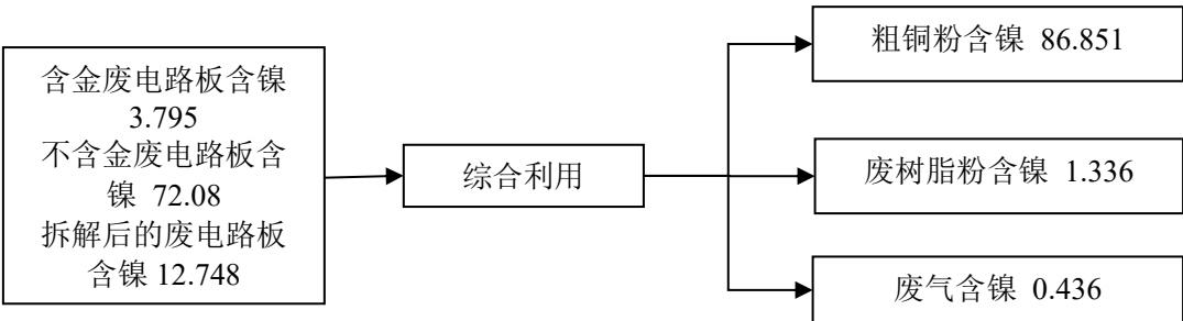
图 3.4-5 废电路板破碎分选生产线镍元素平衡示意图 单位：t/a
