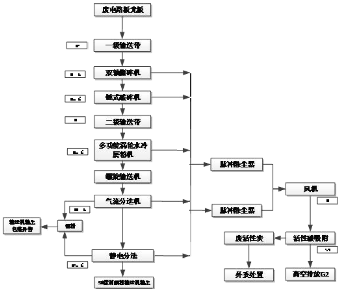
图 3.4-5 废电路板破碎分选生产线工艺流程及产污环节图
