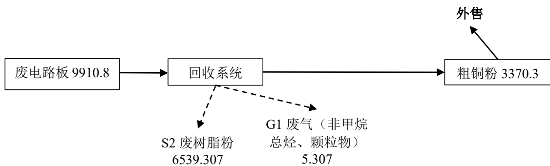
图 3.4-6 废电路板破碎分选生产线物料平衡图 (单位 t/a)
