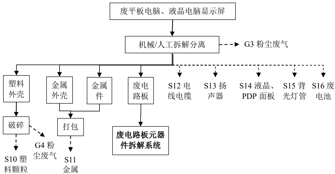
图 3.4-13 平板电脑、液晶电脑显示屏拆解工艺流程及产污环节图
