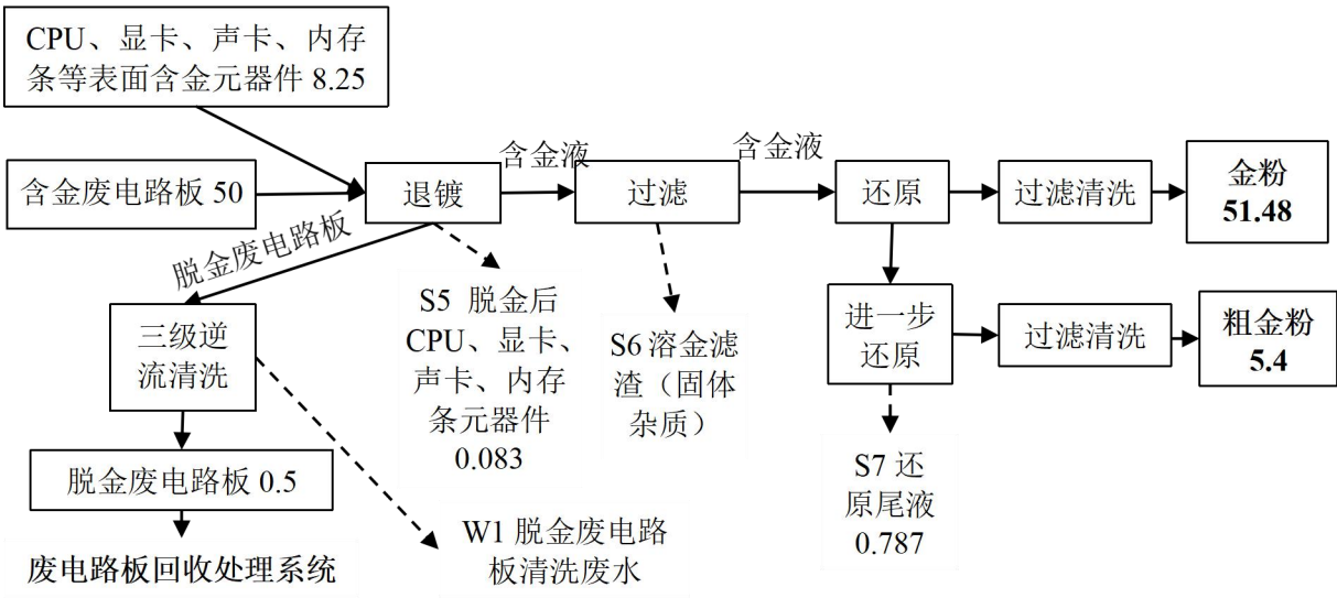
图 3.4-4 含金废物退镀系统金平衡图（单位 kg/a）
