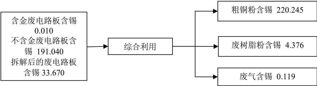
图 3.4-5 废电路板破碎分选生产线锡元素平衡示意图 单位：t/a
