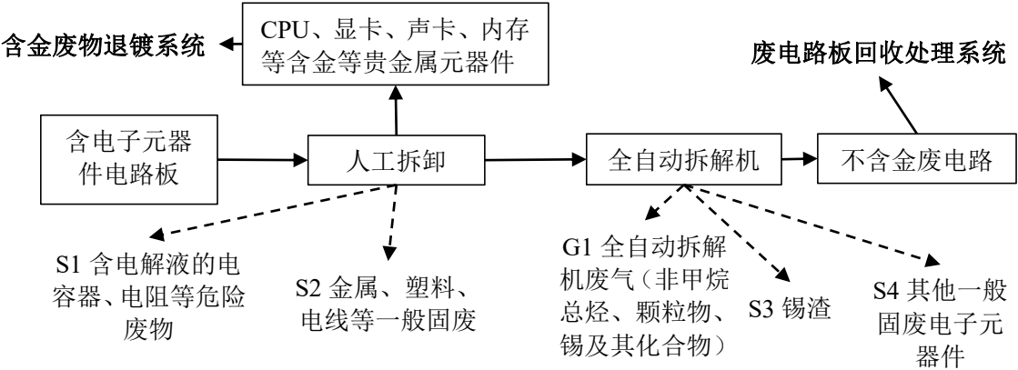
图 3.4-1 废电路板元器件拆解系统工艺流程及产污环节图
