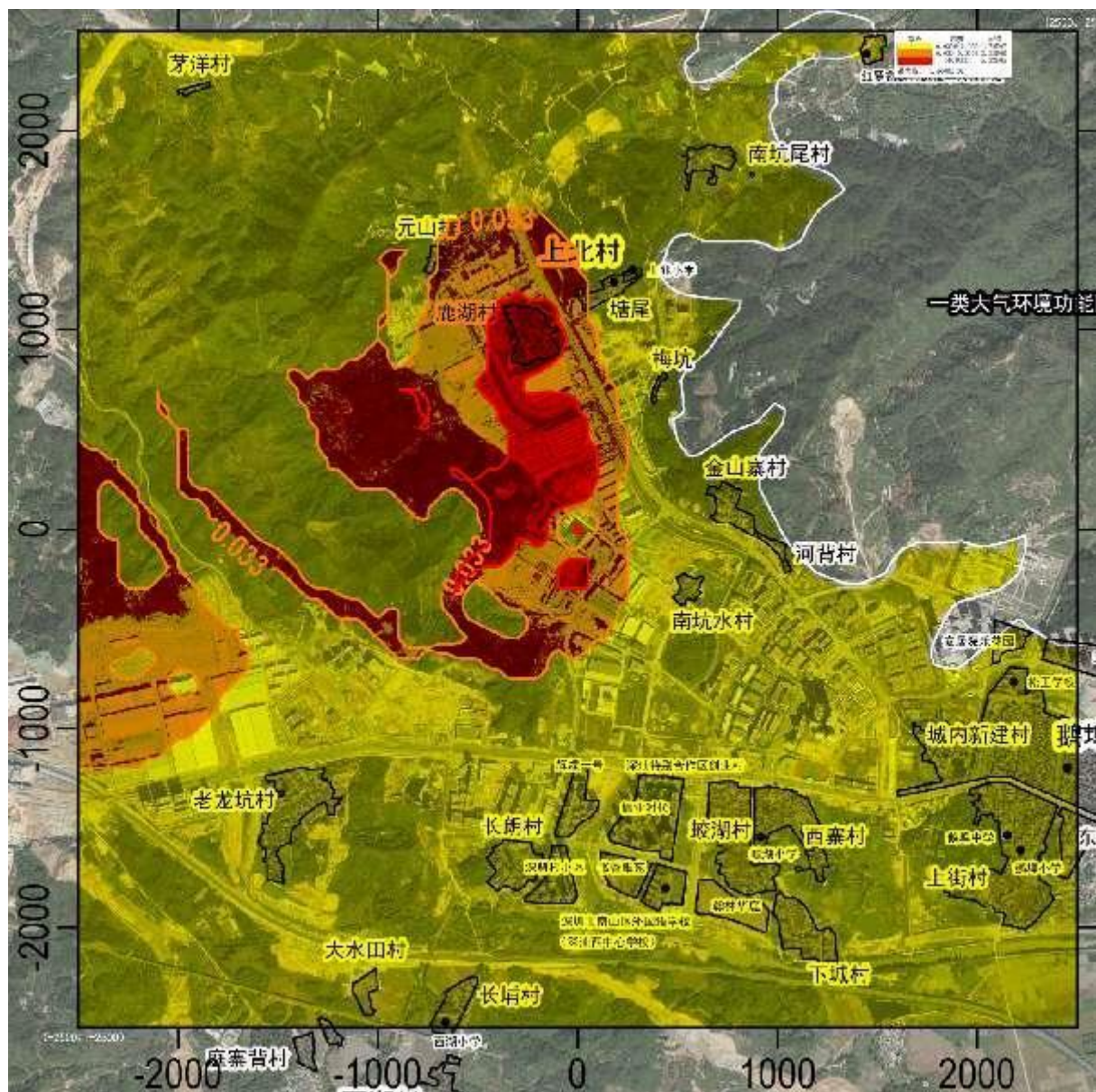
图 5.1-9 PM 10 叠加现状浓度后年平均质量浓度分布图( \mu\text{g}/\text{m}^3 )
