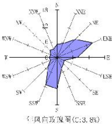
图 5.1-1 惠东风向玫瑰图（静风频率 3.8%）
