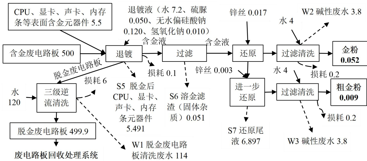
图 3.4-4 含金废物退镀系统物料平衡图（单位 t/a）
