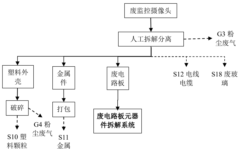
图 3.4-14 废监控摄像头拆解工艺流程及产污环节图
