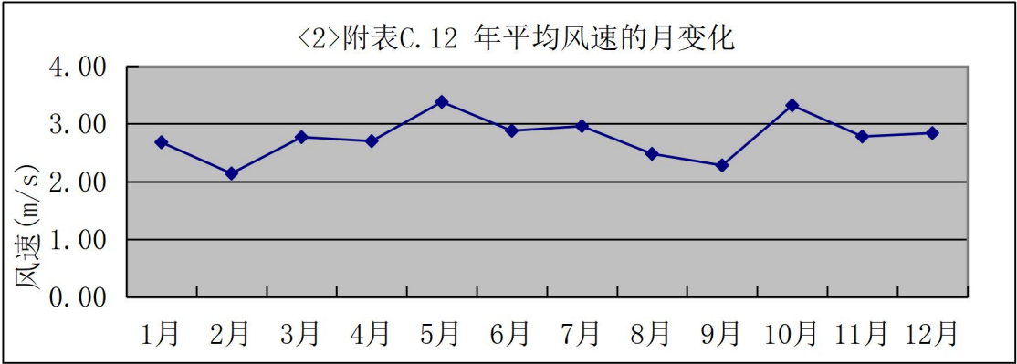
图 5.1-3 2021 年平均风速月变化图
