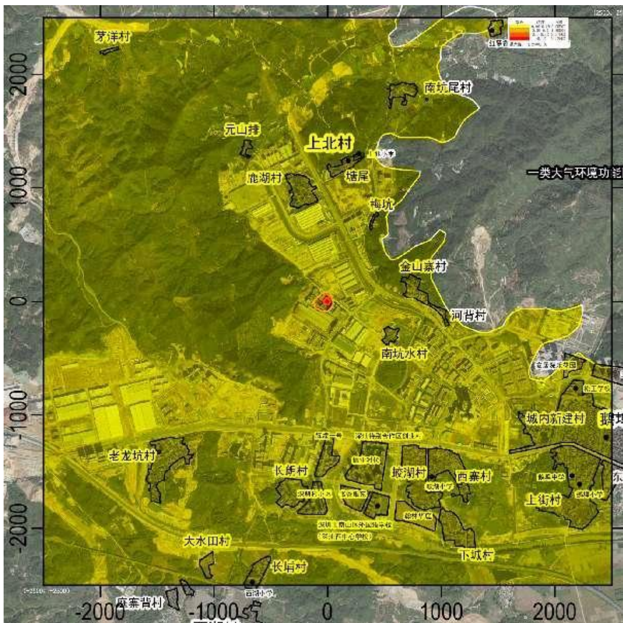
图 5.1-11 TSP 叠加年均质量浓度分布图( \text{mg}/\text{m}^3 )
